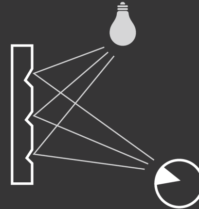
refleksijski hologram
