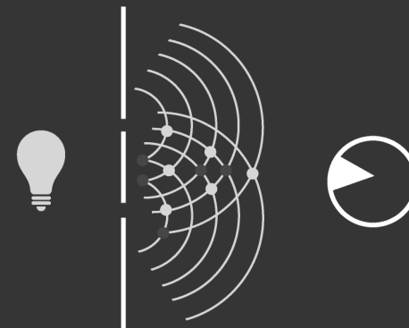
transmisijski hologram
